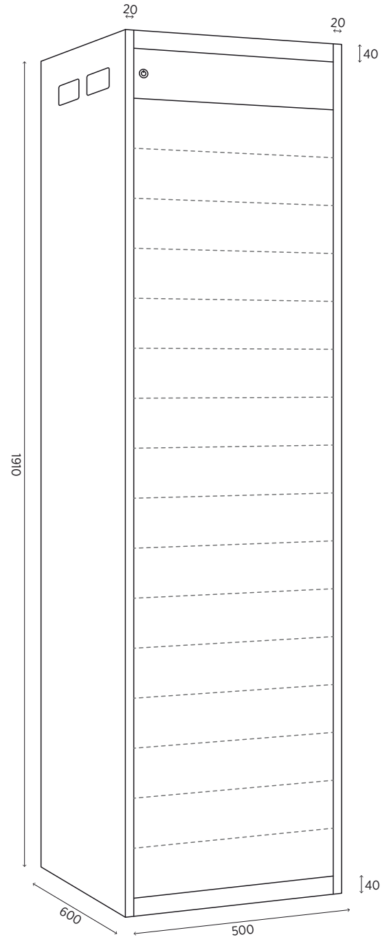
TAMAÑOS DE PUERTAS SERIE 500
