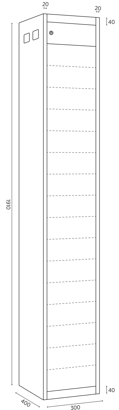
TAMAÑOS DE PUERTAS SERIE 300
