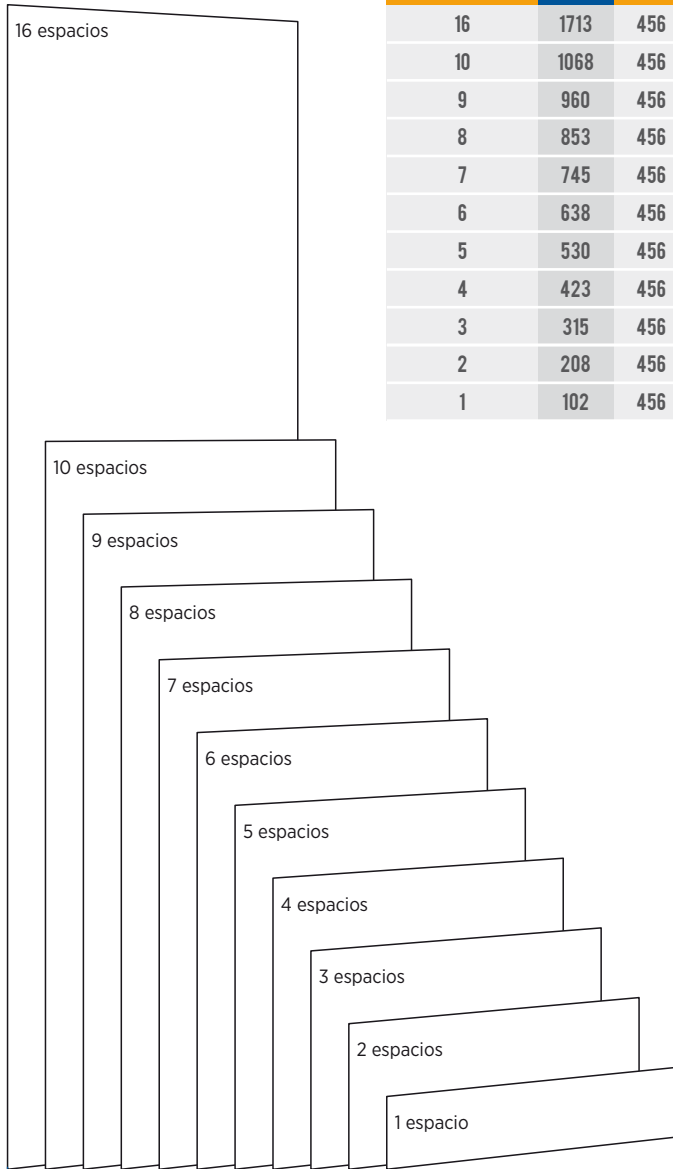
TAMAÑOS DE PUERTAS SERIE 500
